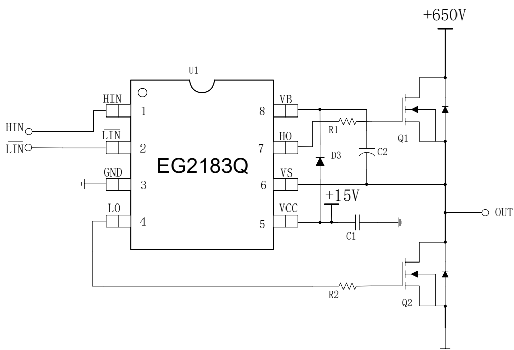
图 6-1. EG2183Q 典型应用电路图
