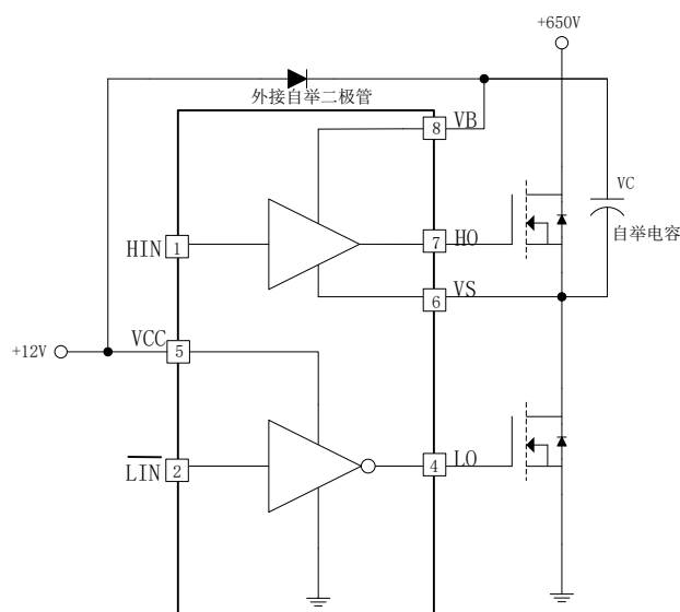
图 8-3. EG2183Q 自举电路结构
