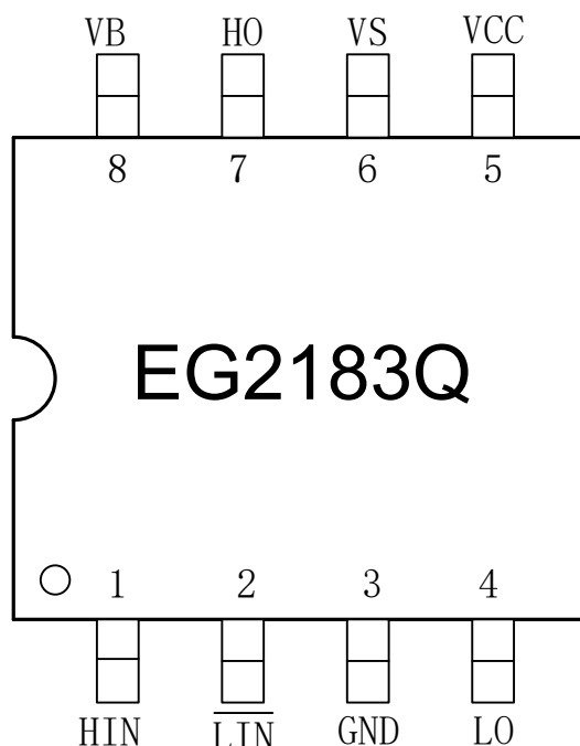
图 4-1. EG2183Q 管脚定义
