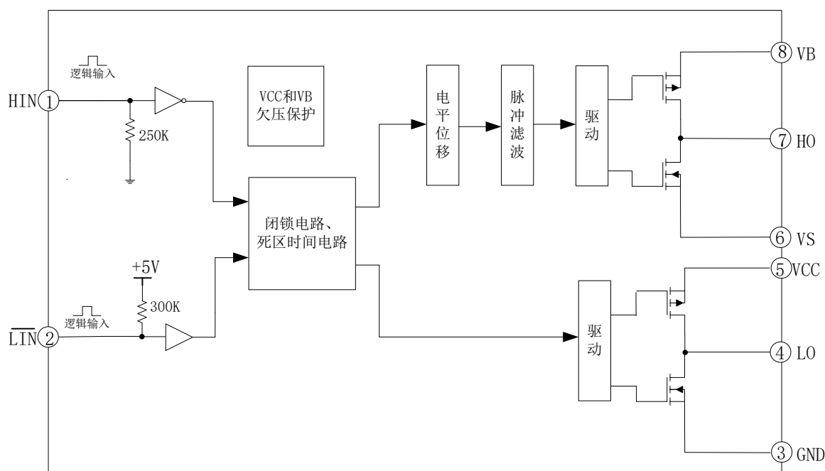
图 5-1. EG2183Q 内部电路图
